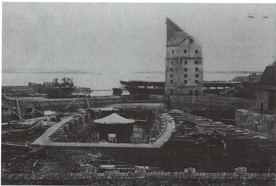
Mastkranen och dockorna. Mastkranen användes för att lyfta de kollosala linjeskeppsmasterna på plats i fartygen eller som på bilden avmastning. På detta ca 140 år gamla fotografi, signerat fotograf Karl Karlsson, Karlskrona, se vi just ett av de sista gamla linjeskeppen, framför kranen.
